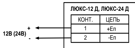
Рис.1. Схема подключения.
